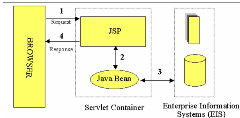
Figura 3.1 Esquema funcionamiento tecnología JSP
